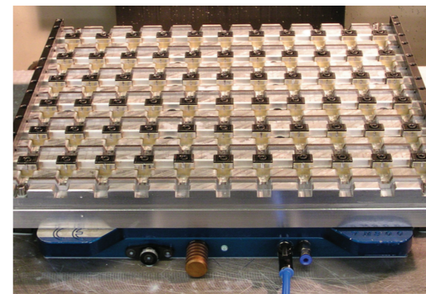
*VM300 真空吸盤 (45175) 和 VM300 (45130)
