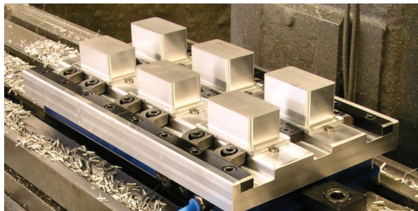
*真空吸盤 VM100 (45375) 和治具板 (45325)
