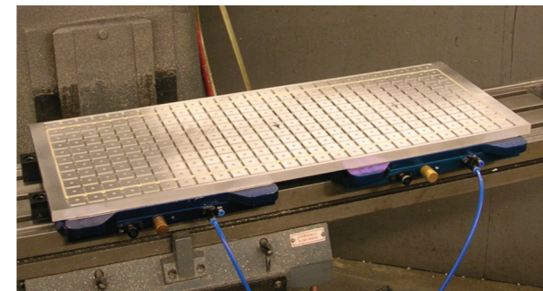
*VM300 真空吸盤2個
