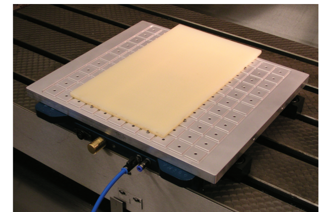
*工件置於橡膠條上且向下推以製造真空準備加工。
