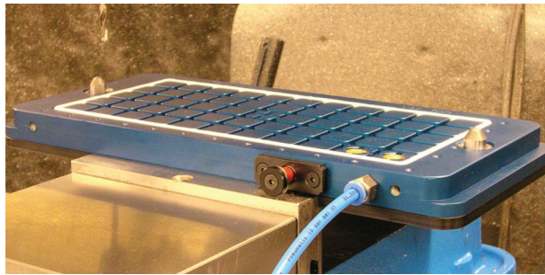
*虎鉗夾持真空吸盤 VM100
